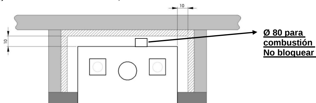
Imagen 3. Revestimiento del espacio de inserción – paredes combustibles y aislamiento
