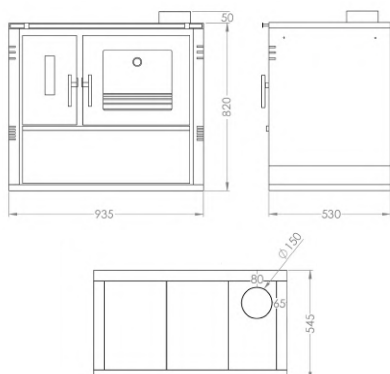
Saída de fumos do lado direito ou do lado esquerdo (opcional)
