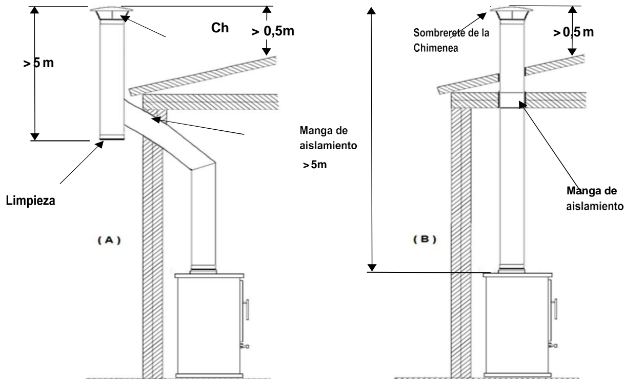
Figura 1. Ejemplo de instalación de chimenea
