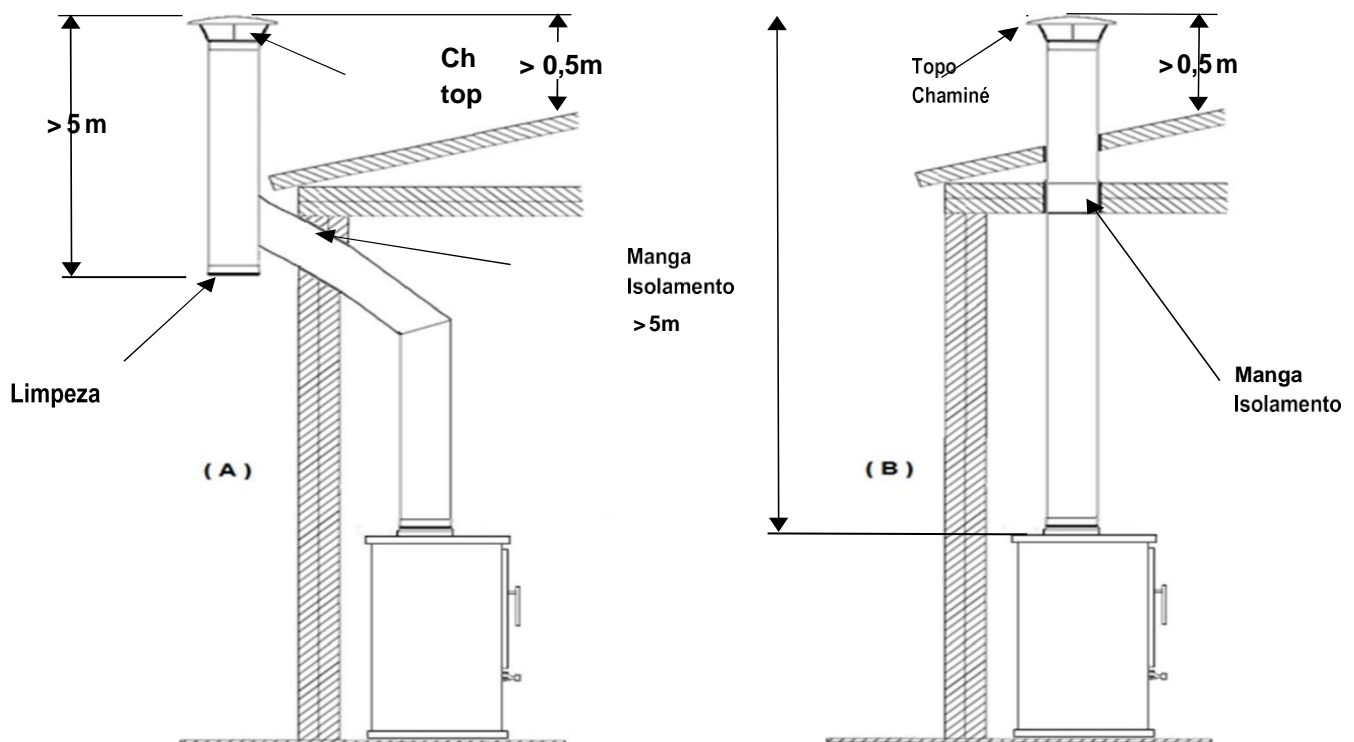
Figura 1. Exemplo de instalação de chaminé
