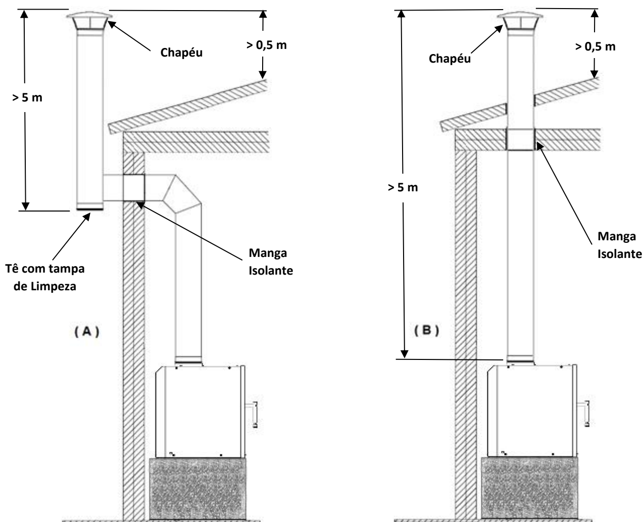
Figura 4. Diagrama da ligação do recuperador à chaminé
