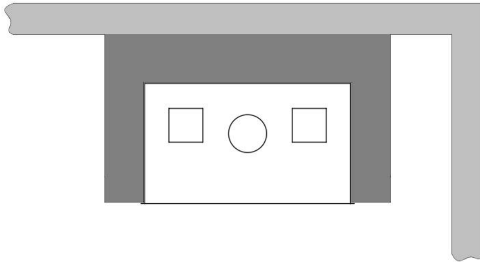
Figura 6. Revestimento do espaço de inserção – paredes não combustíveis com boa resistência térmica
