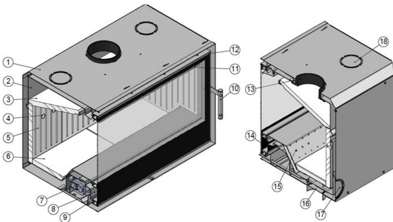
Figura 3. Recuperador de calor Elos Evolux
