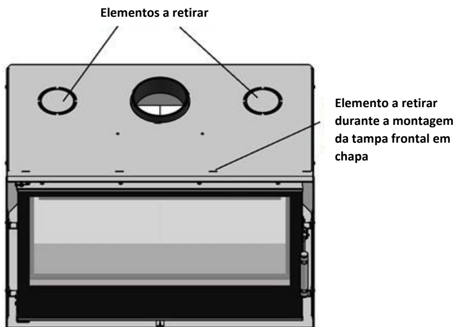
Figura 8. Locais de corte antes de montar as boquilhas para o sistema de distribuição de ar quente.
