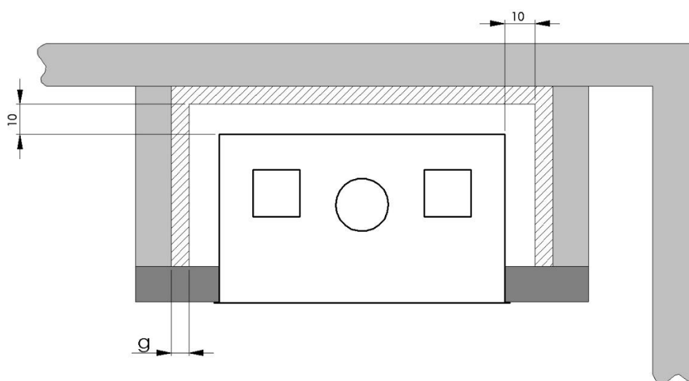
Figura 5. Revestimento do espaço de inserção – paredes combustíveis e isolamento
