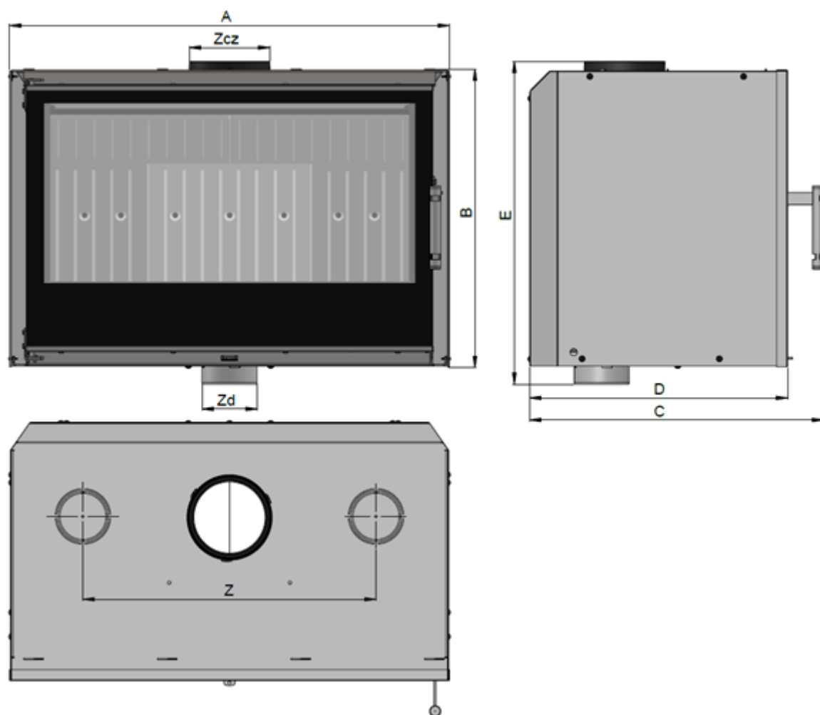
Figura 2. Dimensões tipo dos recuperadores de calor Elos Evolux
